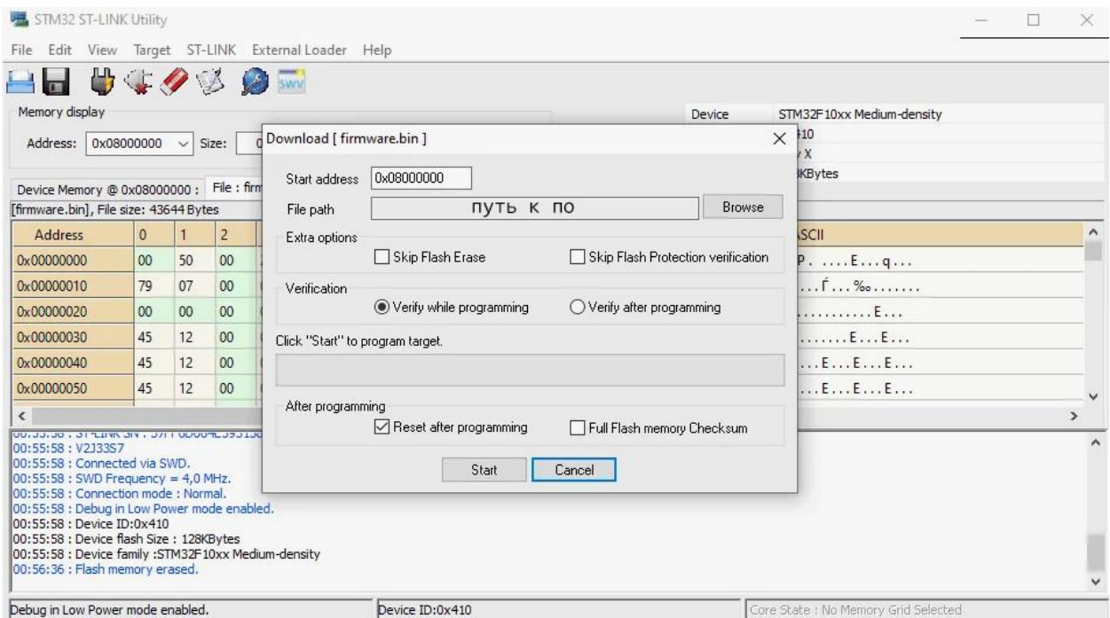
Рис. 6 установка ПО
